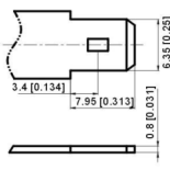
Клемма F2
