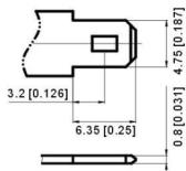
Клемма F1
