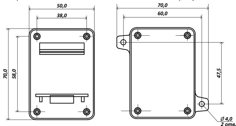
Рисунок 3. Монтажные основания с замком на рейку DIN (слева) и проушинами.
