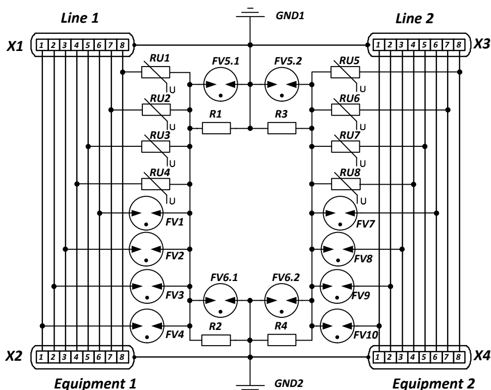
Рис.2 Схема принципиальная Commeng 2-FEP
