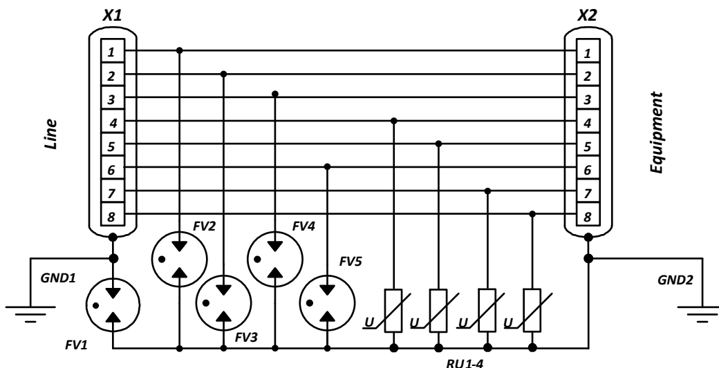
Рис.2 Схема принципиальная.
